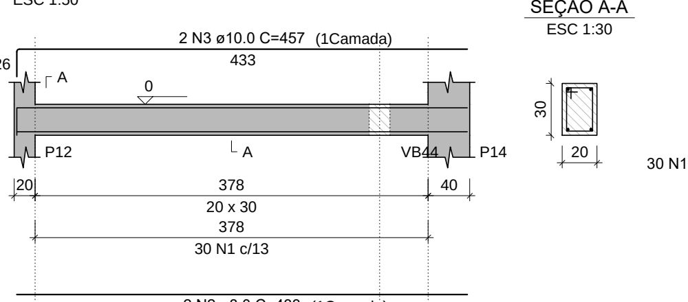
VB3 (20 x 30)
