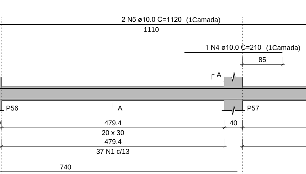
VB17 (20 x 30)
