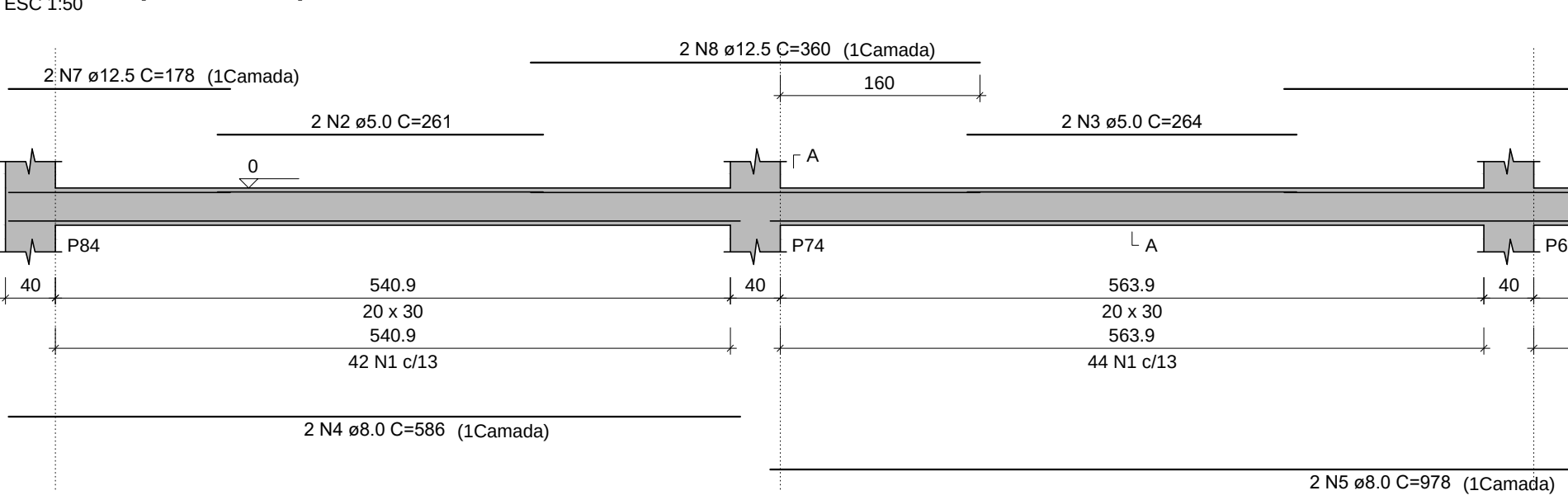
VB29 (20 x 30)
