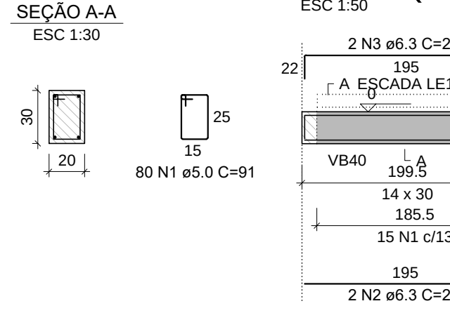
VB33 (20 x 30)
