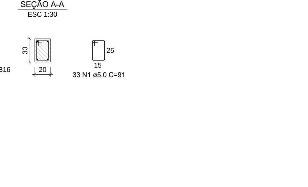
VB39 (20 x 30)
