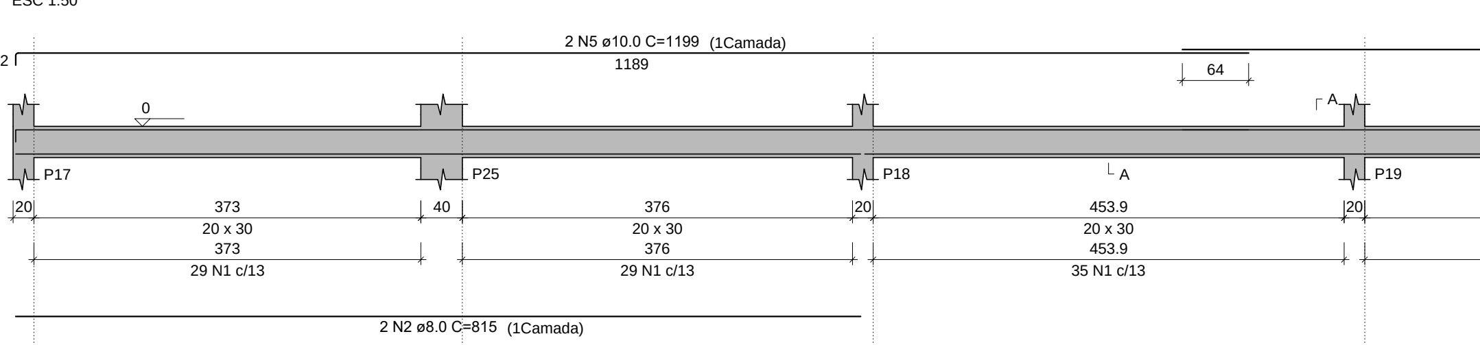
VB10 (20 x 30)
