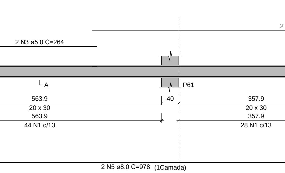
VB29 (20 x 30)
