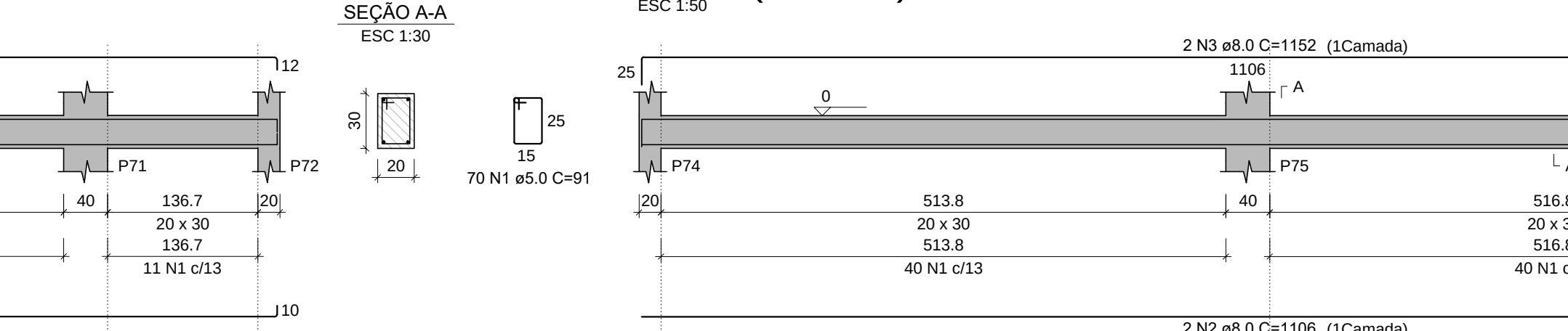
VB33 (20 x 30)
