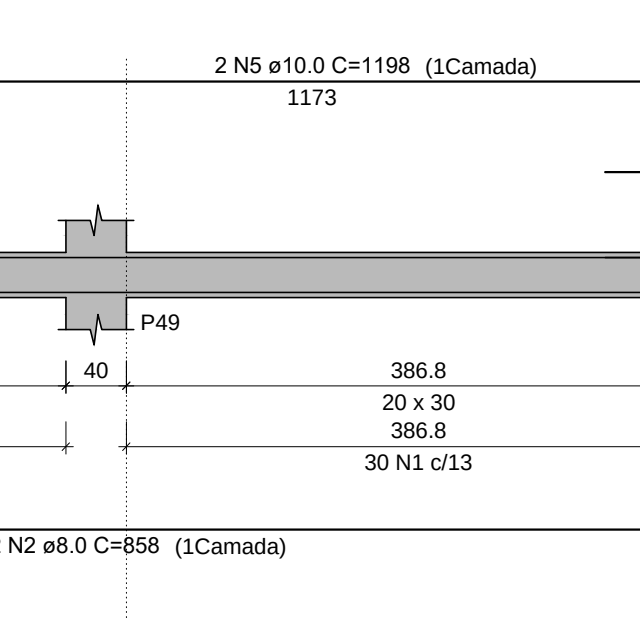
VB20 (20 x 30)
