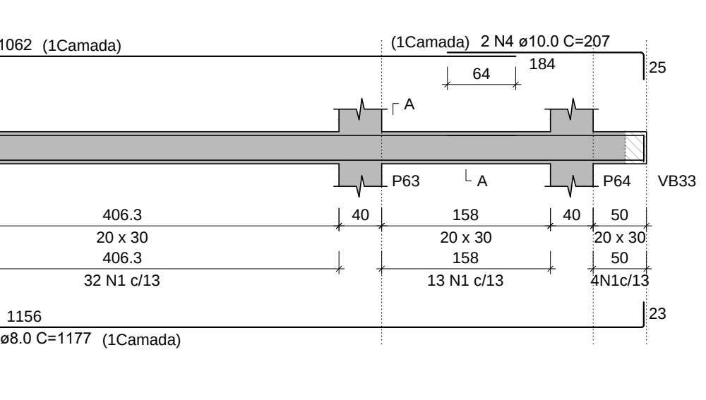
VB20 (20 x 30)
