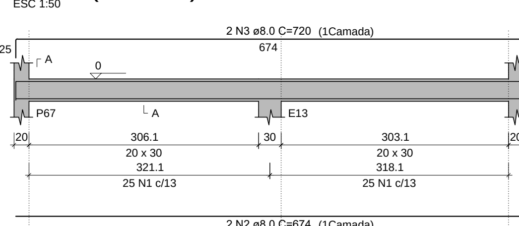
VB24 (20 x 30)
