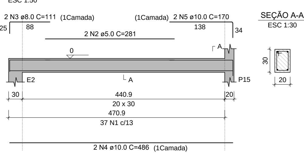
VB8 (20 x 30)
