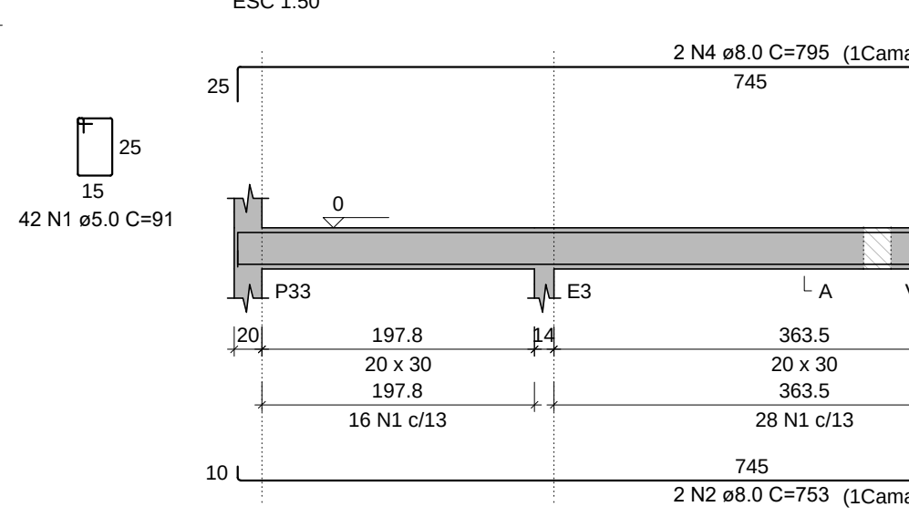
VB9 (20 x 30)
