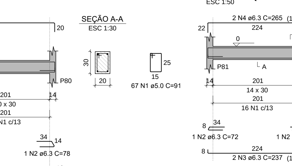
VB26 (14 x 30)
