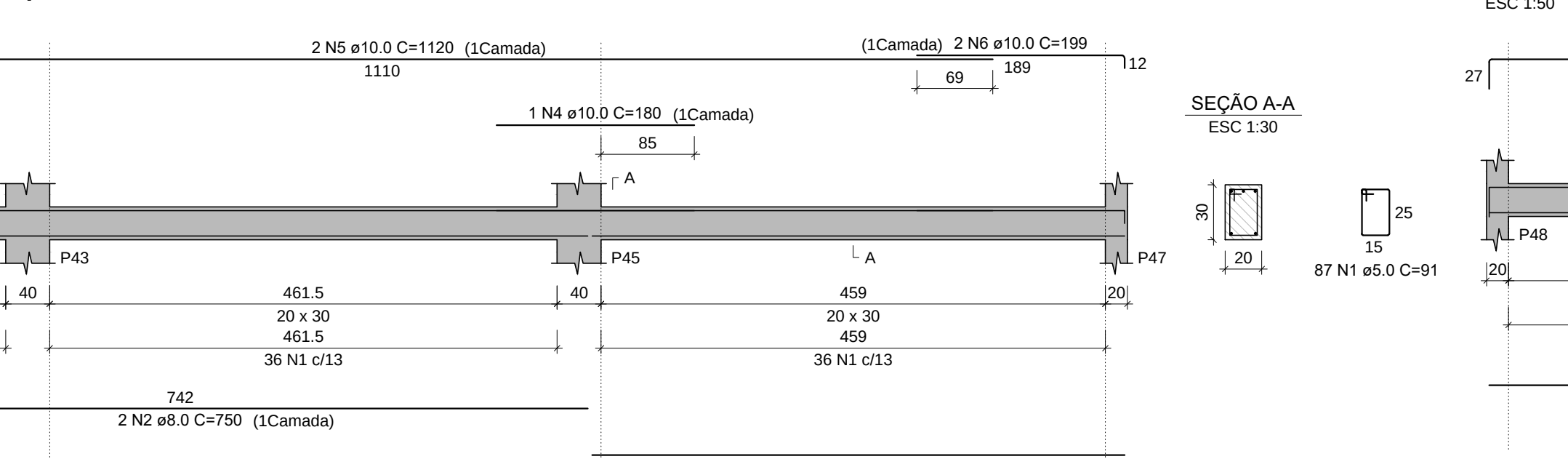
VB18 (20 x 30)
