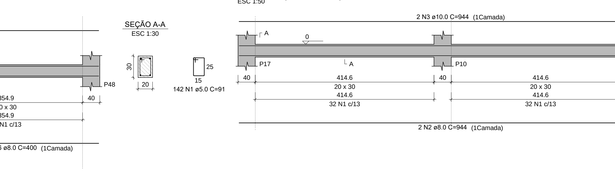
VB39 (20 x 30)
