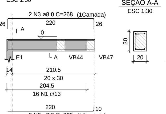
VB2 (20 x 30)
