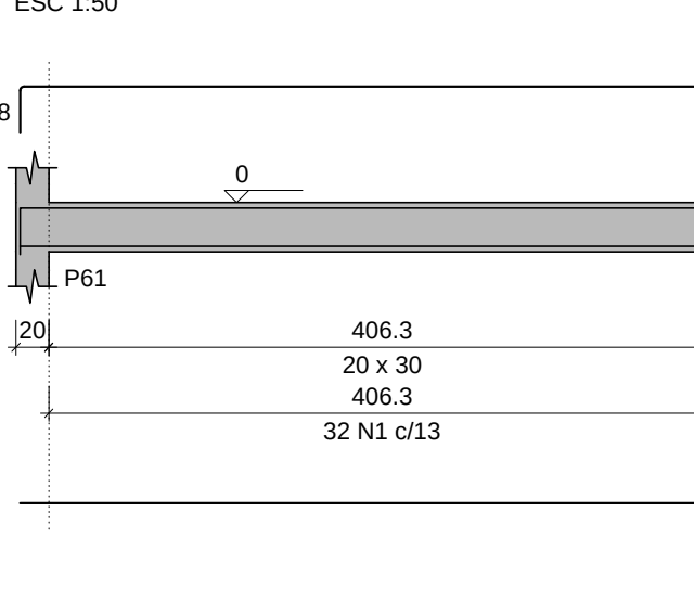
VB20 (20 x 30)
