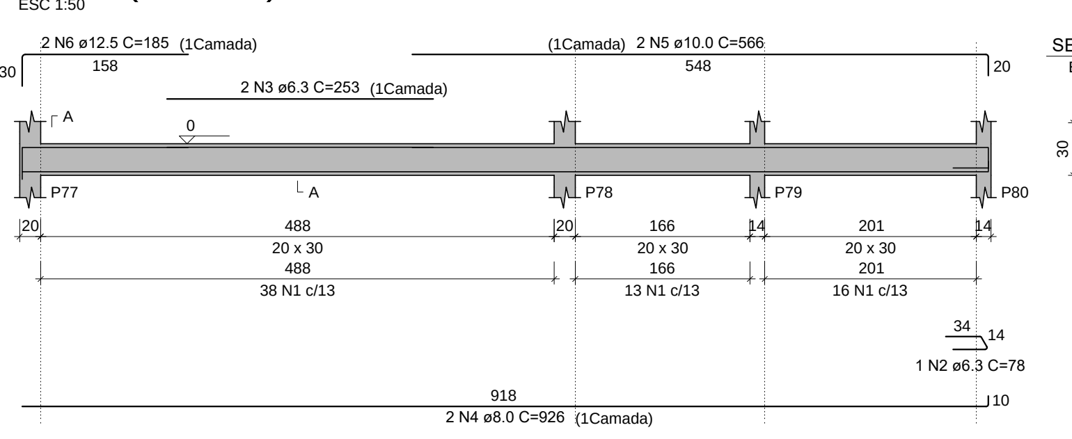
VB24 (20 x 30)
