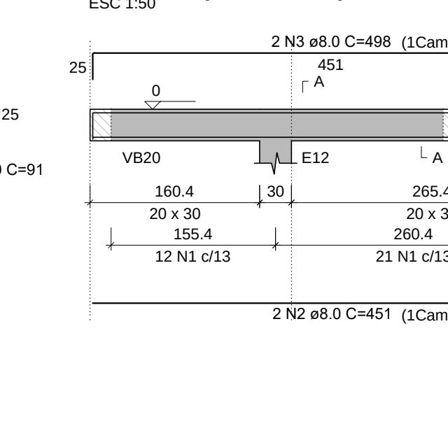
VB39 (20 x 30)
