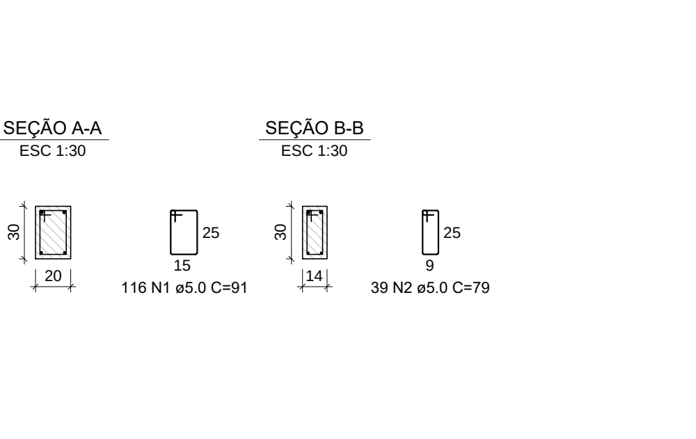
VB33 (20 x 30)
