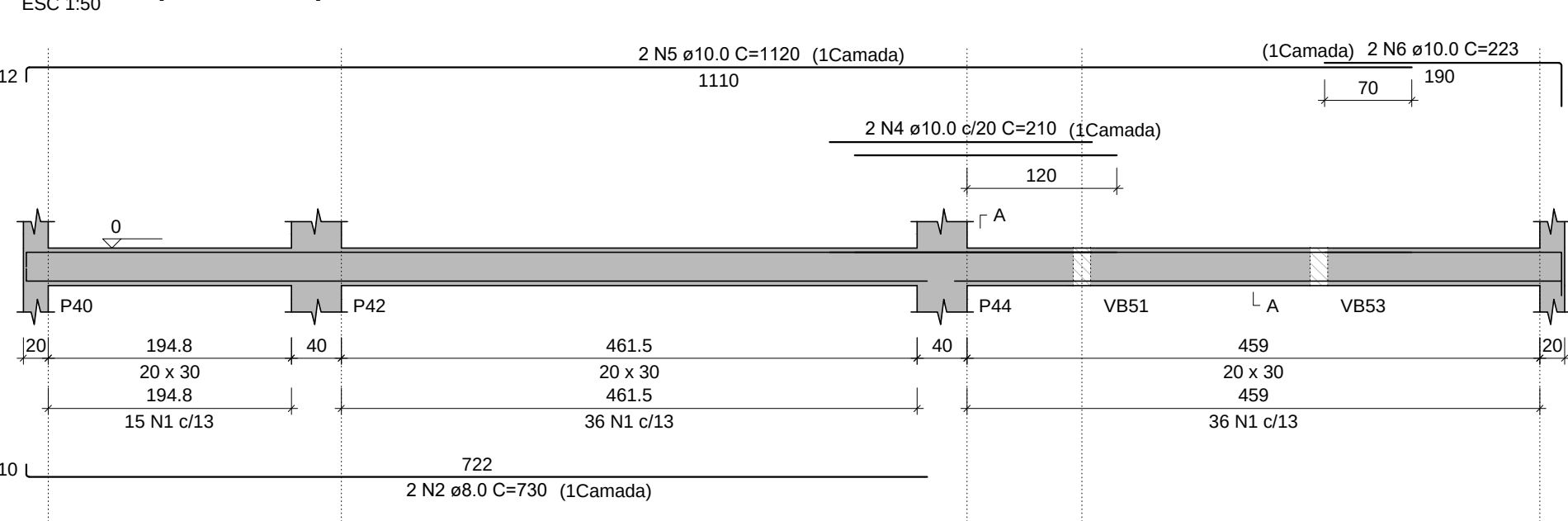
VB16 (20 x 30)
