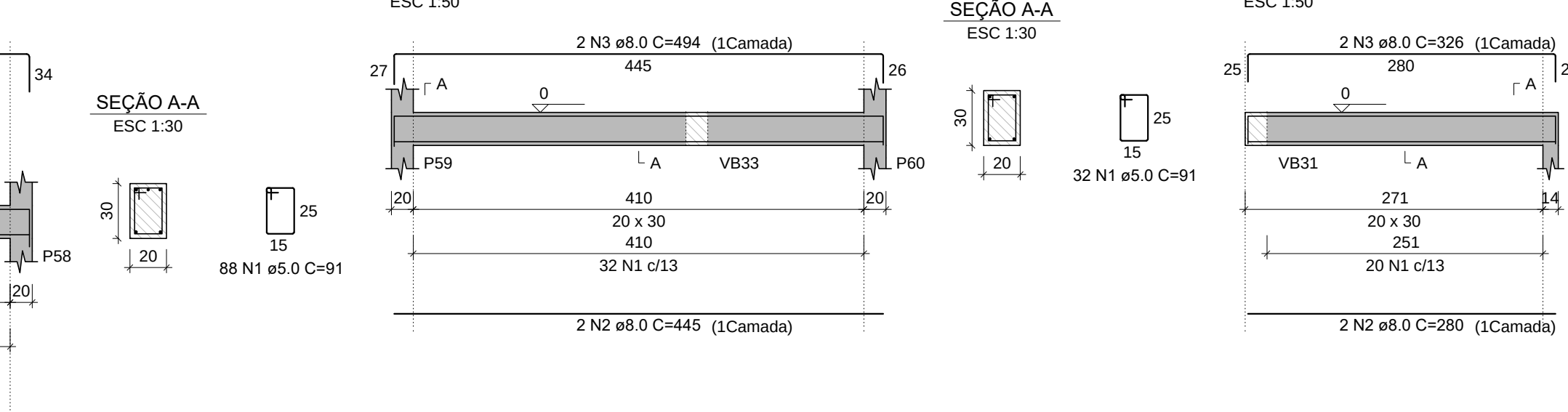
VB18 (20 x 30)
