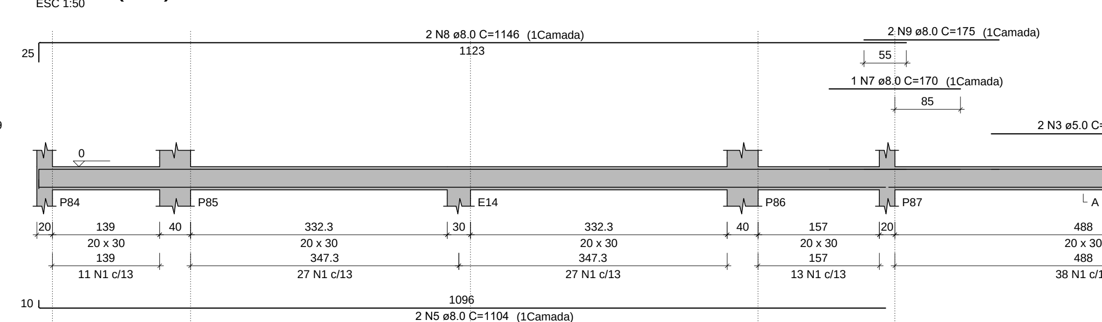
VB33 (20 x 30)
