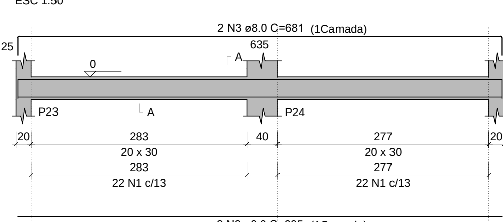
VB5 (20 x 30)
