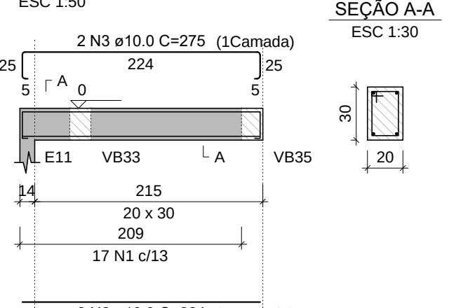
VB16 (20 x 30)
