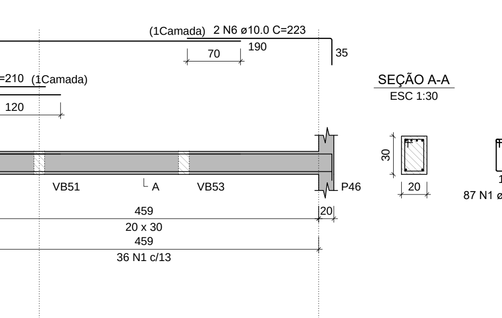
VB17 (20 x 30)
