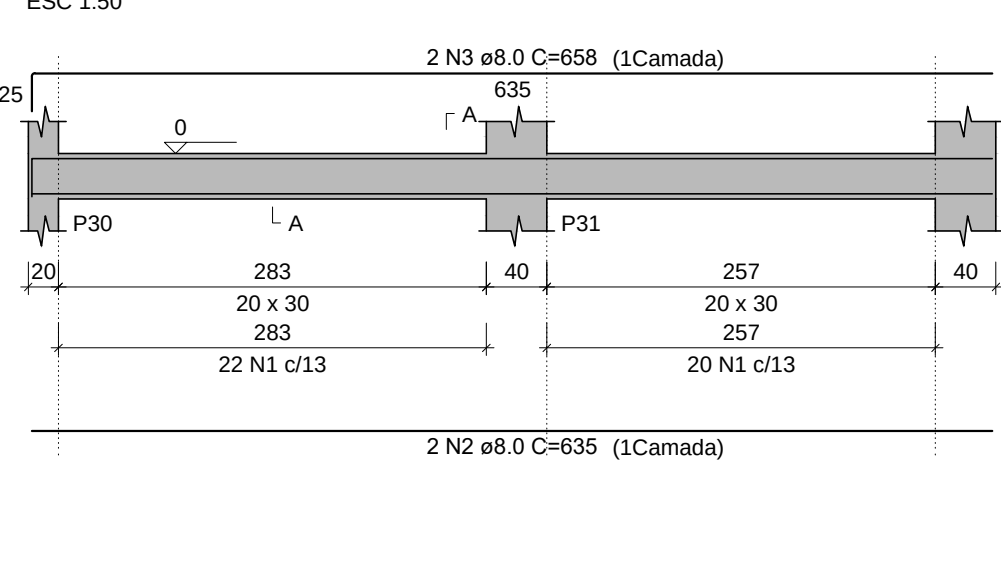
VB8 (20 x 30)
